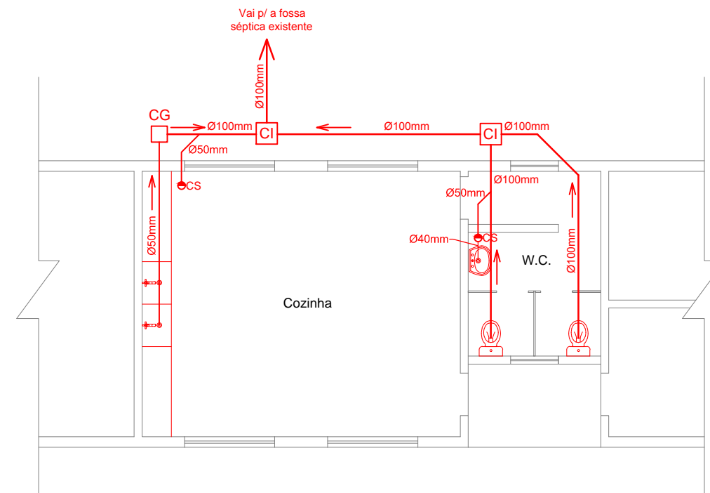
Planta Hidro-Sanitária Esc: 1:100
