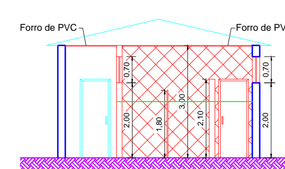
Corte B - B Esc: 1:100
