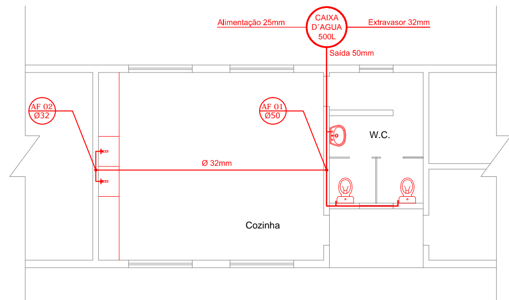
Instalação de Água Fria Esc: 1:100
