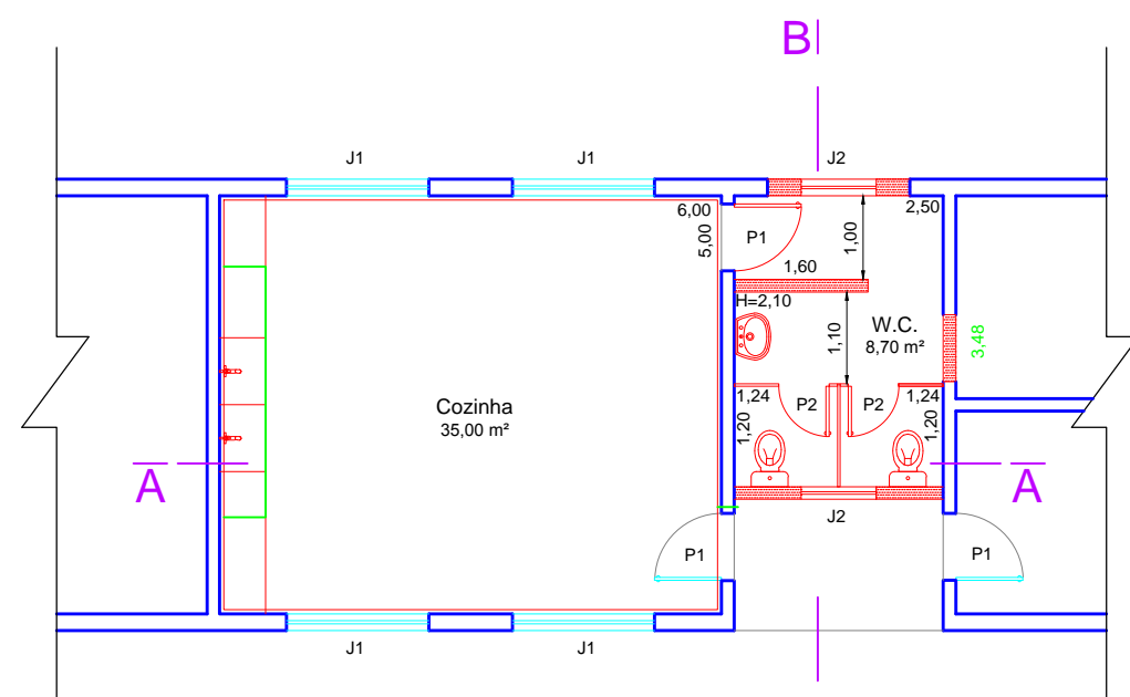
Planta Baixa à Executar Esc: 1:100
