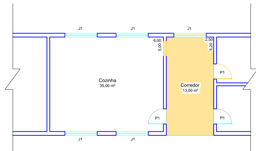
Planta Baixa Existente Esc: 1:100
