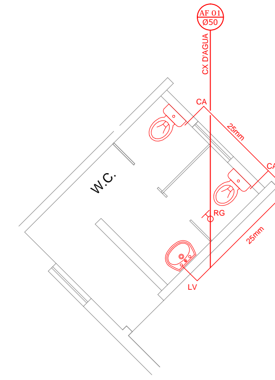
Isométrica do W.C. Esc: 1:75
