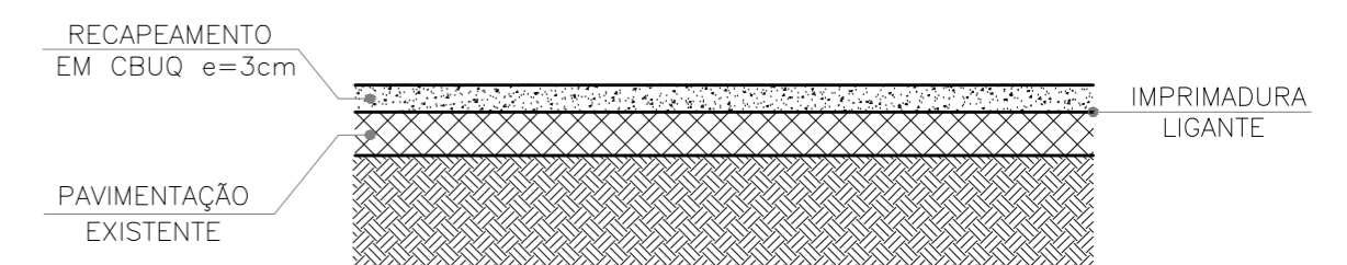
CORTE ESQUEMÁTICO - Recapeamento sem escala
