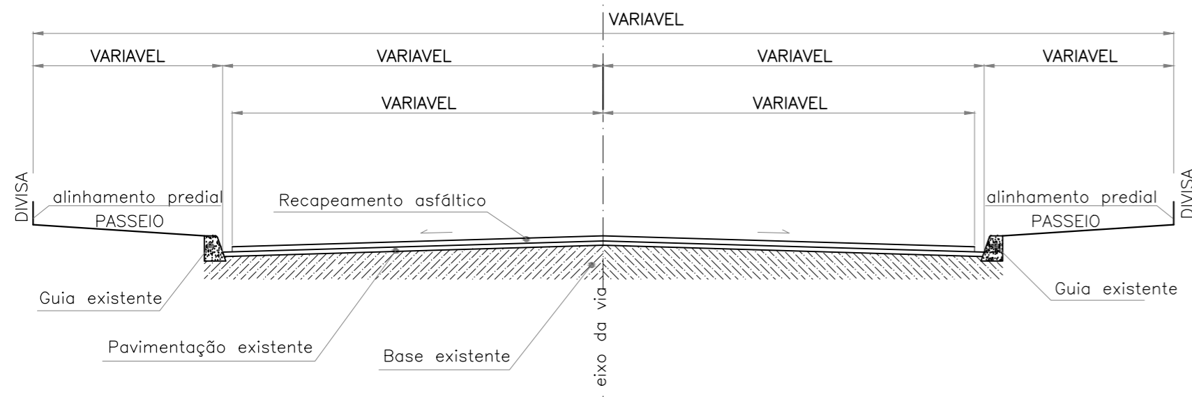
DETALHE - Seção Transversal sem escala
