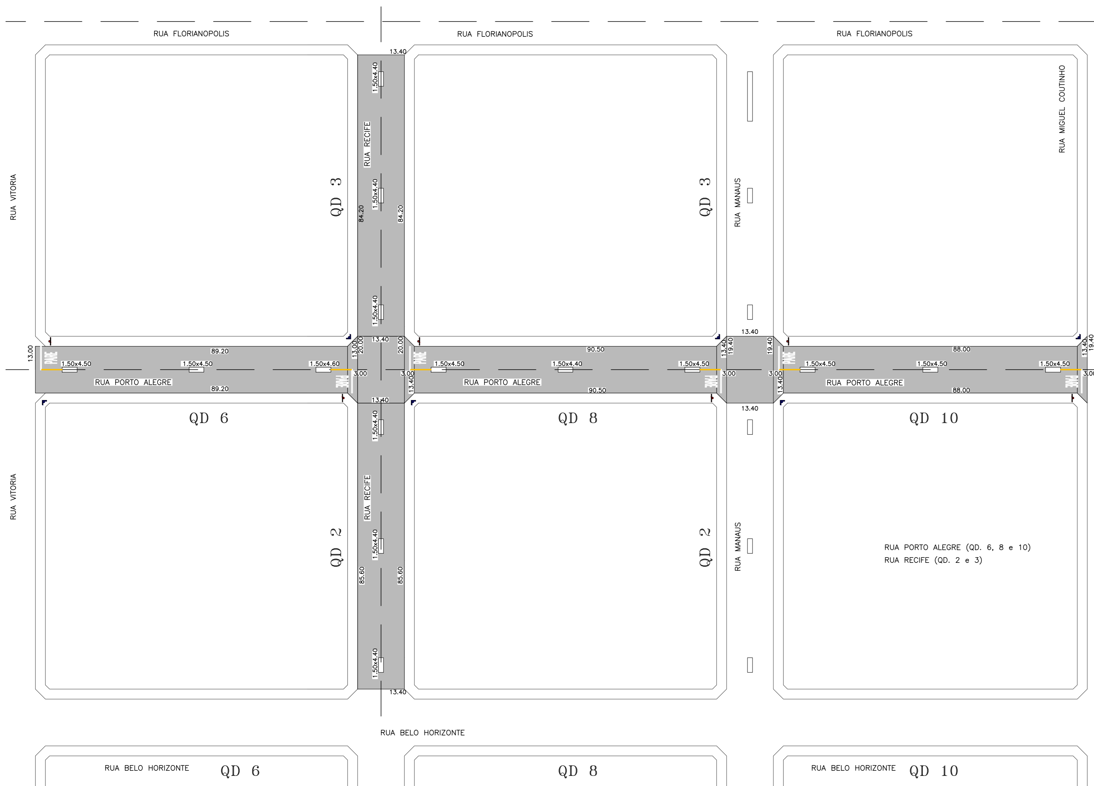
PLANTA - Recapeamento escala 1:750 (m)
