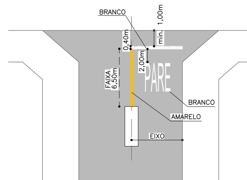
DETALHE: Pintura PARE sem escala
