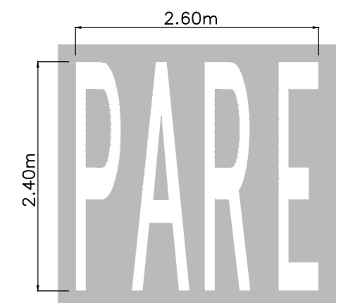
DETALHE - Parada Obrigatória Inscrições no Pavimento Legenda "PARE" sem escala
